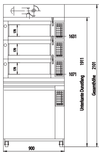
MIWE GVAU mit MIWE condo 3.0608 (Herdhöhe 17 cm)
