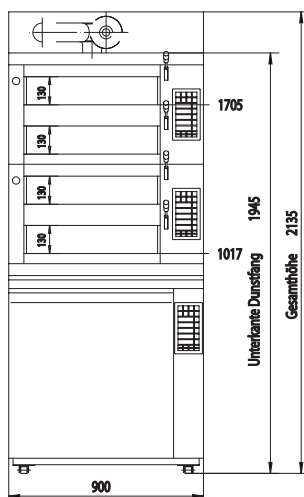
MIWE GVAU mit Doppelbackkammern MIWE condo 4.0608-2D
