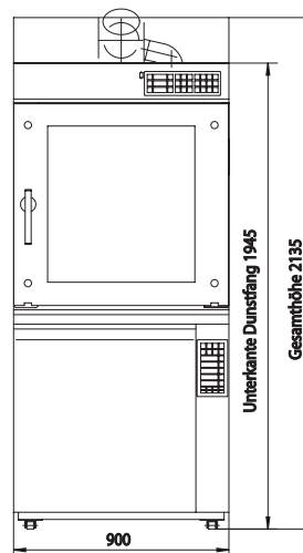
MIWE GVAU mit MIWE aero 8.0604
